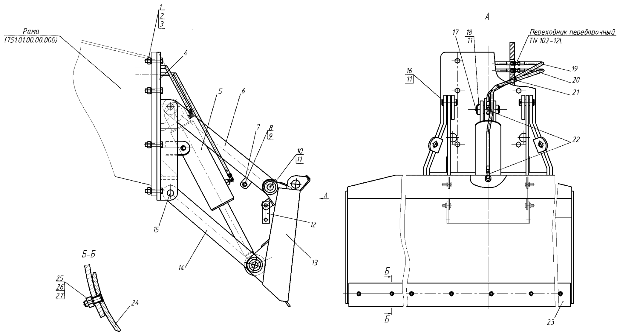
Рис.15 Отвал передний 751.21.00.00.000
