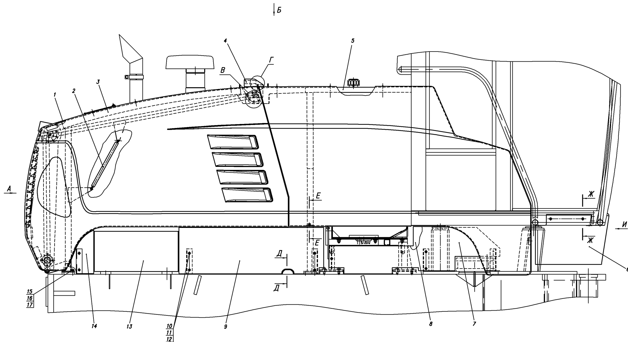
Рис.28.1 Установка облицовок 724.25.00.00.000
