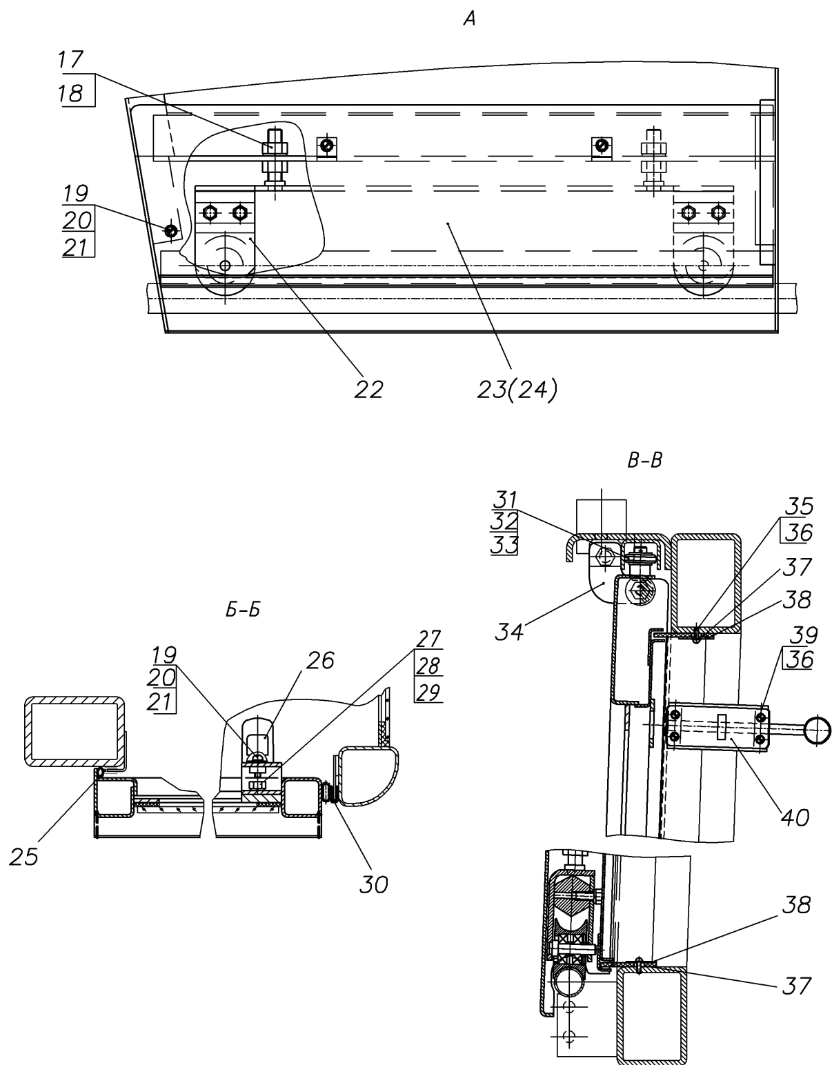
Рис.19.2 Кабина 170.00.00.00.000-01
