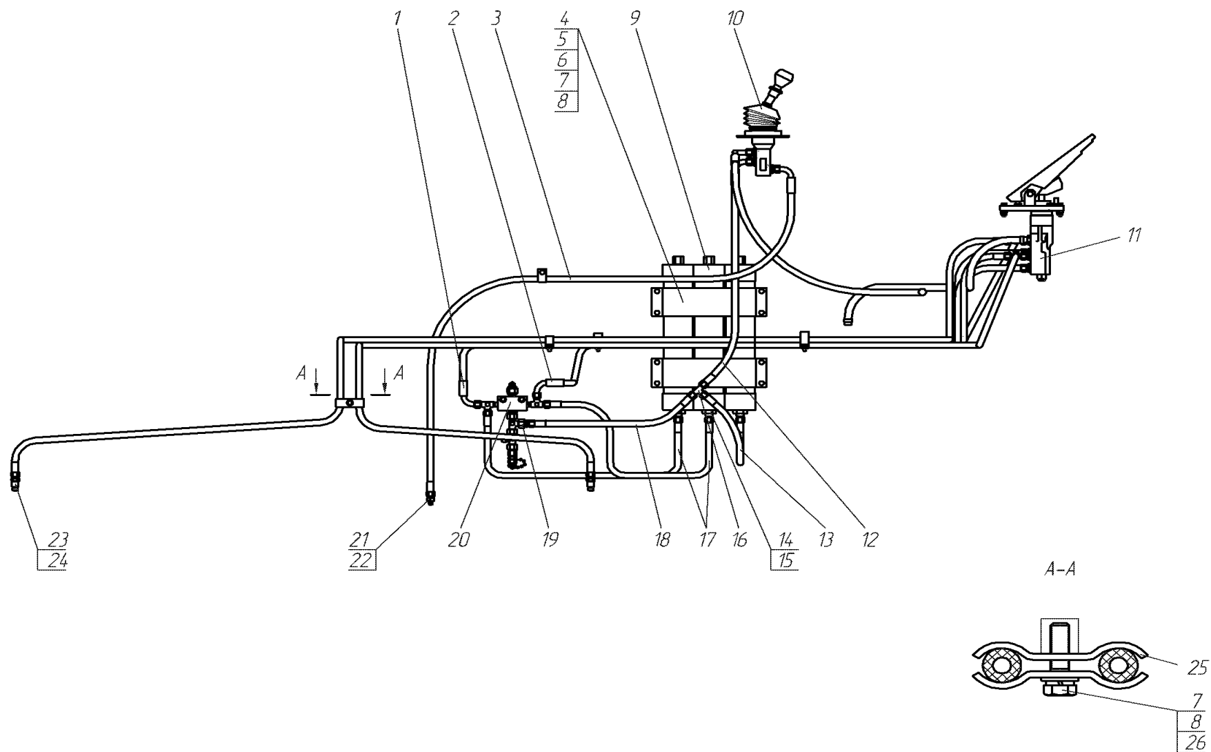
Рис. 35.1 Гидросистема тормозов 257.11.00.00.000
