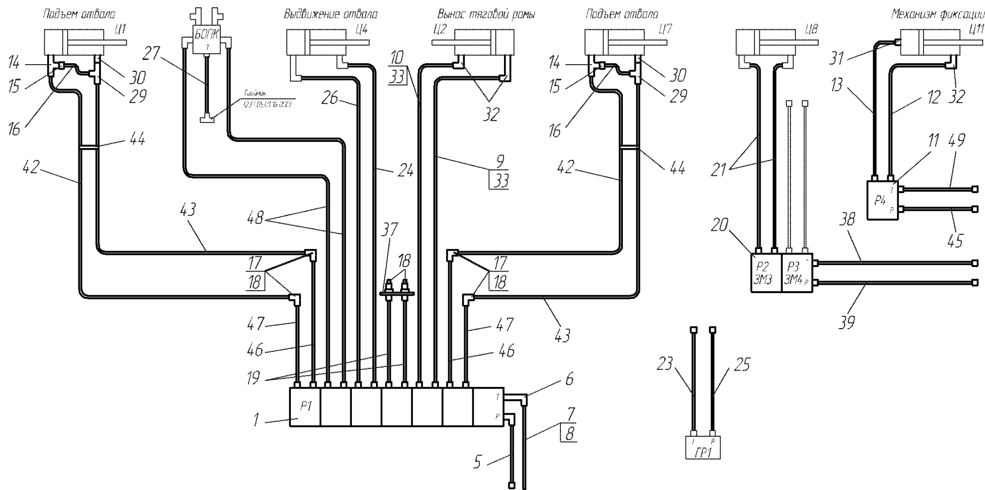
Рис. 33.3 Схема гидравлическая соединений 753.05.03.00.000 Г4
