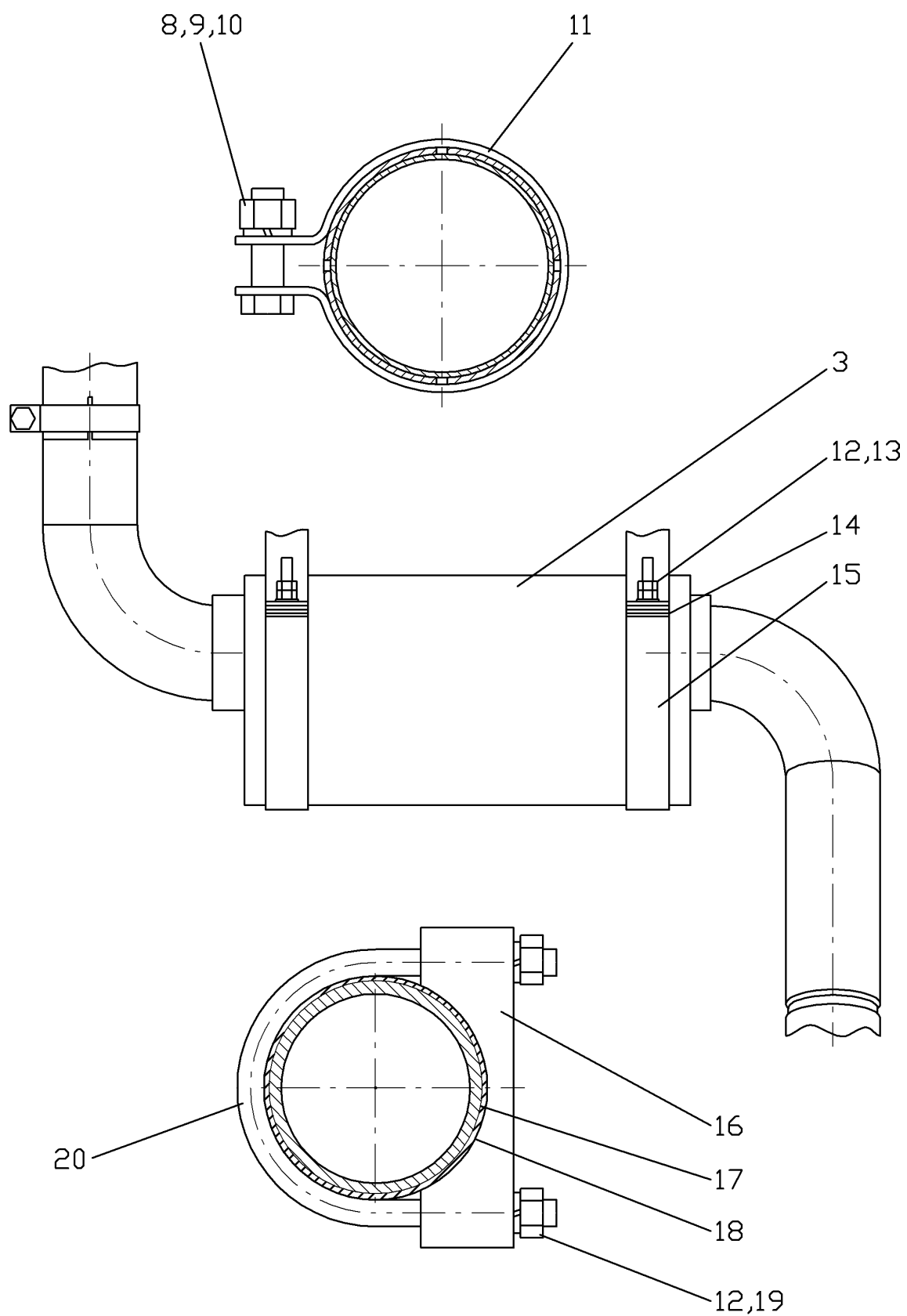
Рис. 47.2 Установка глушителя 724.02.03.00.000
