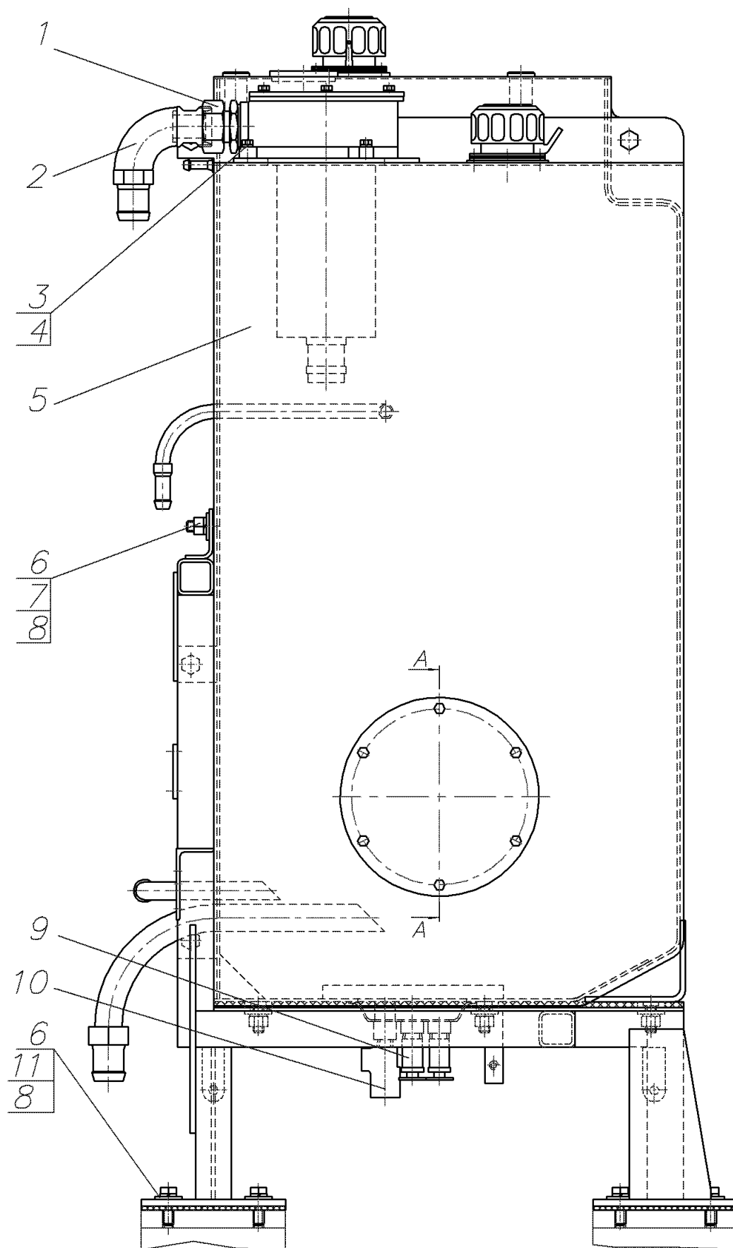
Рис.14.1 Блок баков 724.35.00.00.000
