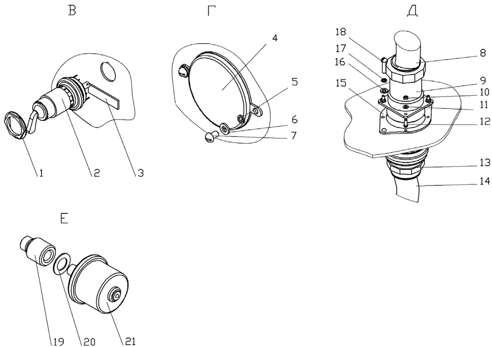
Рис.40.9 Электрооборудование кабины - 112 -
