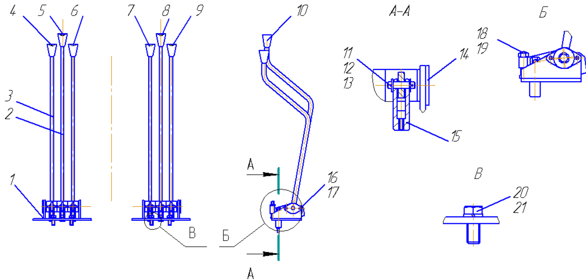
Рис.9 257.04.06.00.000 Установка рычагов
