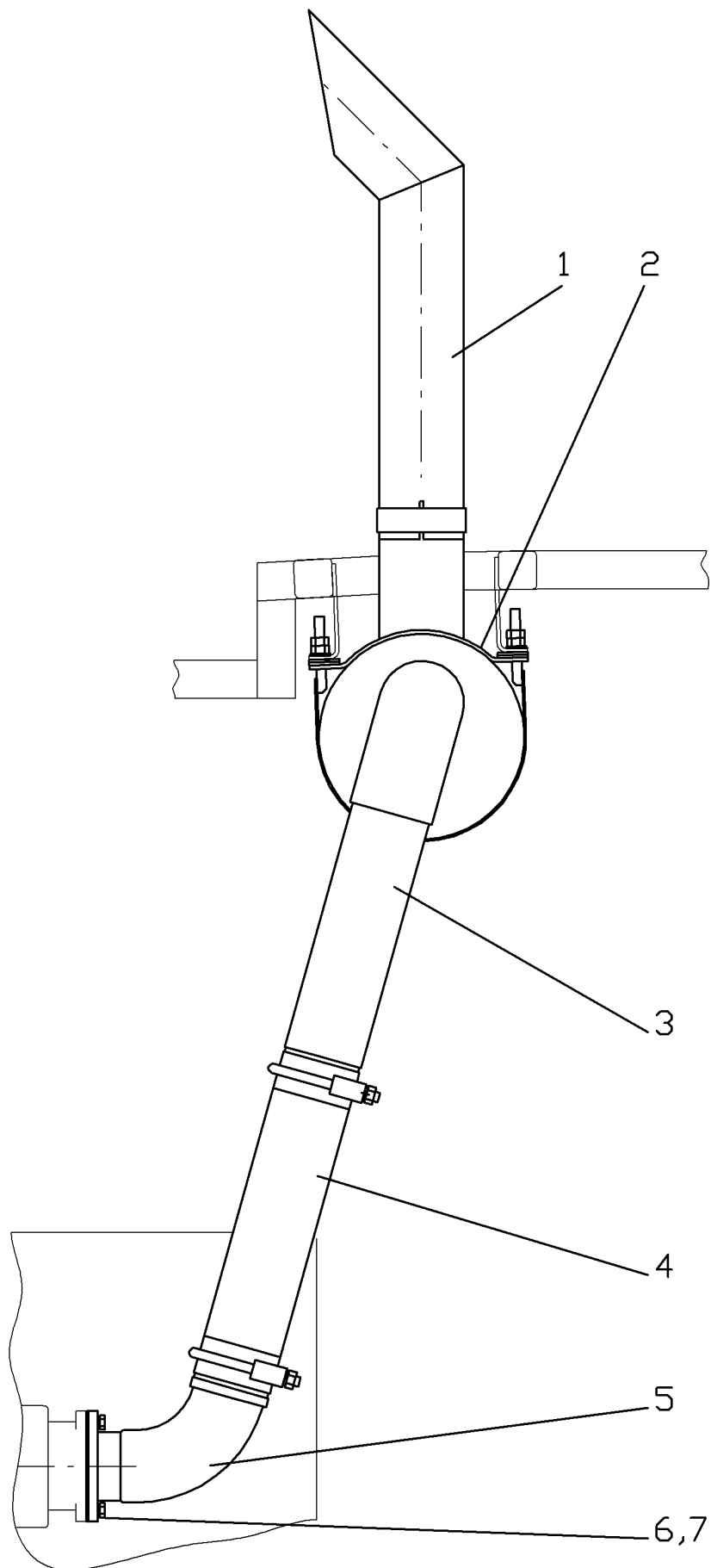
Рис. 47.1 Установка глушителя 724.02.03.00.000
