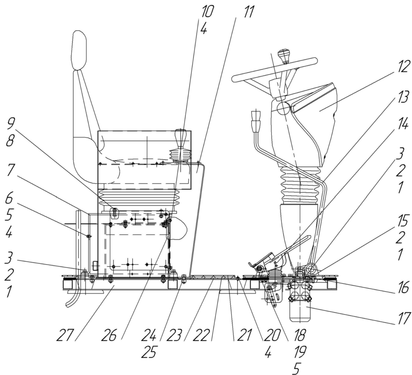
Рис. 4.1 Место рабочее 257.04.00.00.000-01
