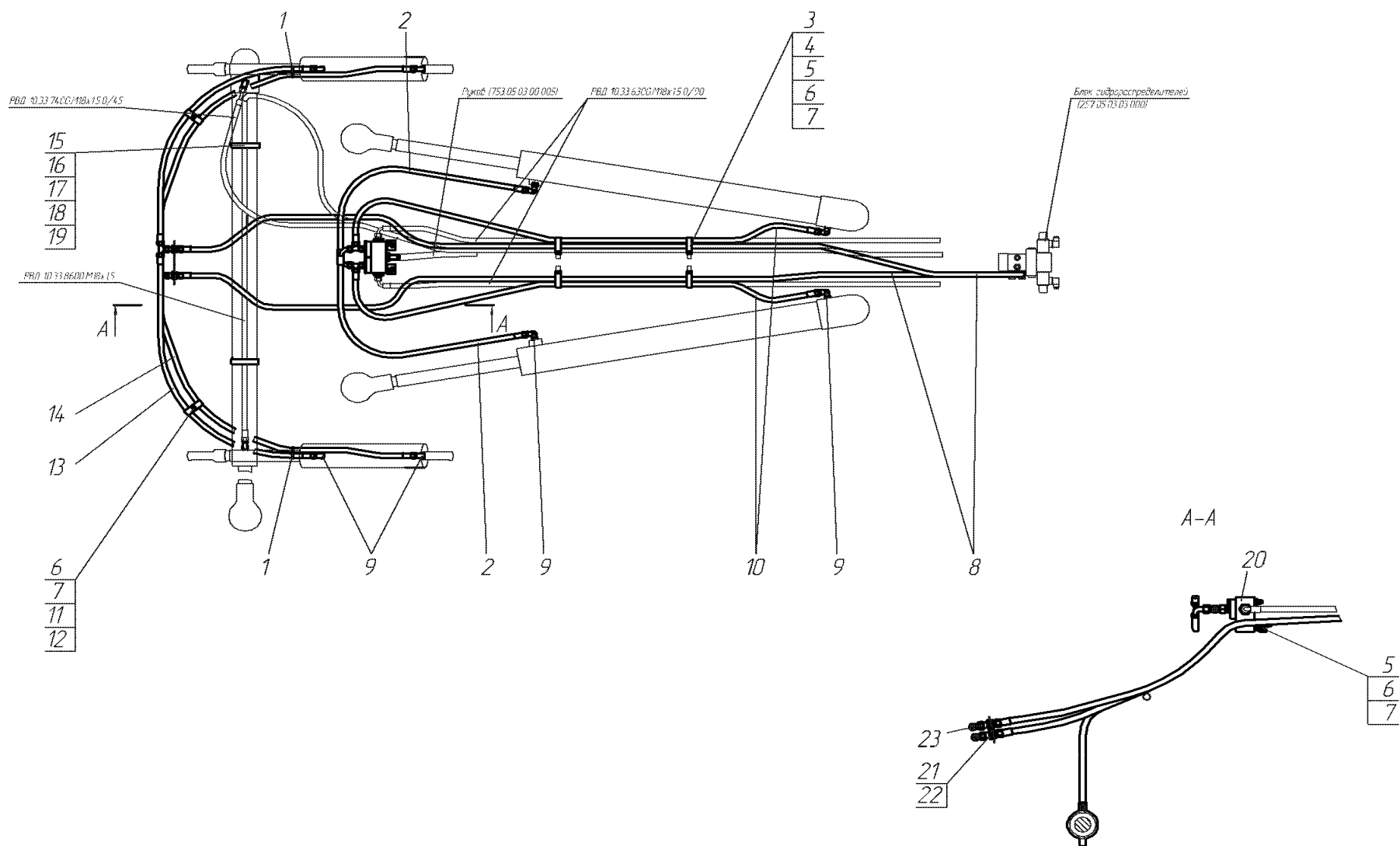
Рис. 32.1 Гидросистема рабочего оборудования 724.05.04.00.000
