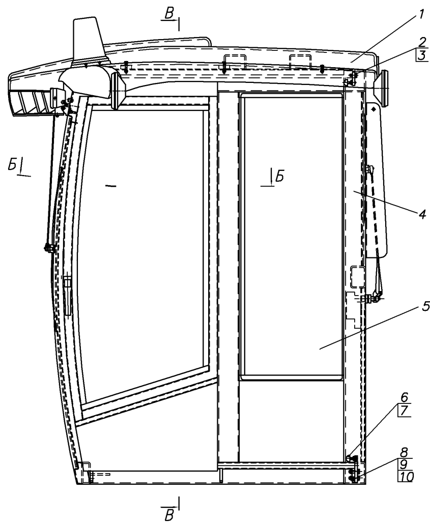
Рис.19.1 Кабина 170.00.00.00.000-01
