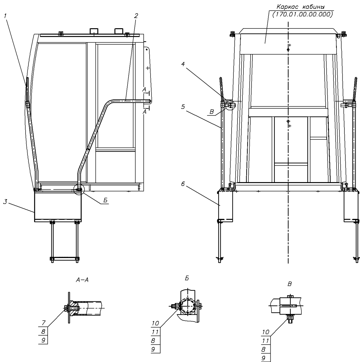
Рис.13 Установка лестниц 724.28.00.00.000
