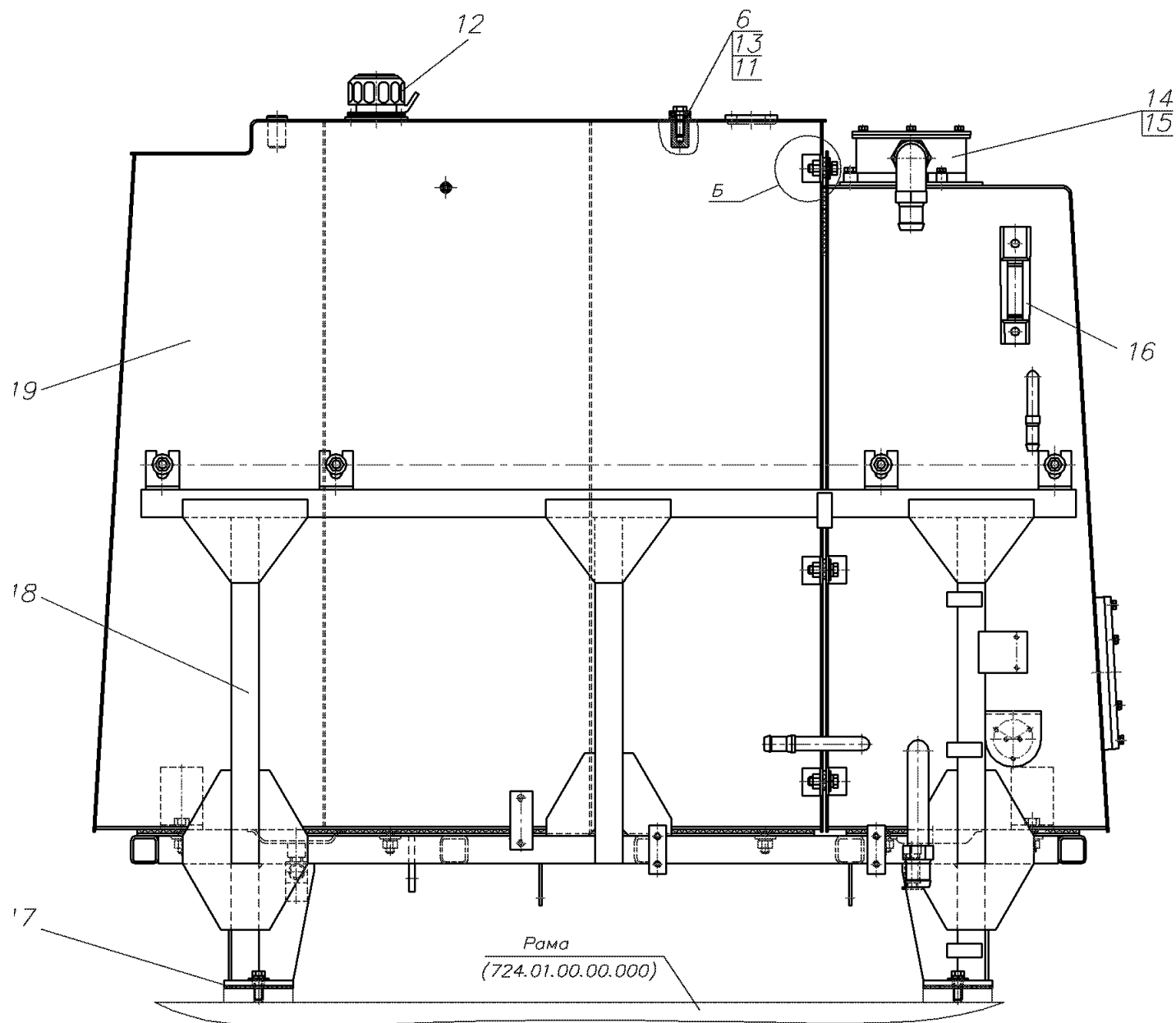
Рис.14.2 Блок баков 724.35.00.00.000 -30-
