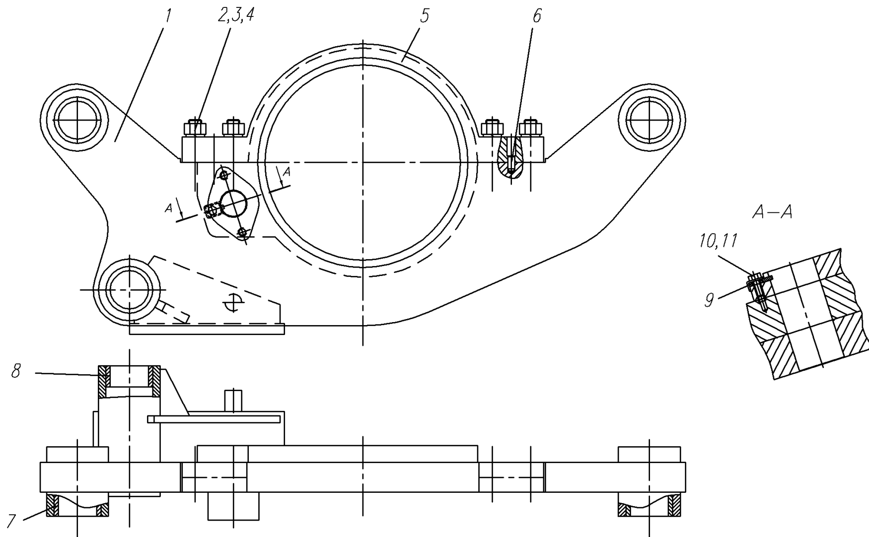
Рис.23 Кронштейн 257.07.03.00.000
