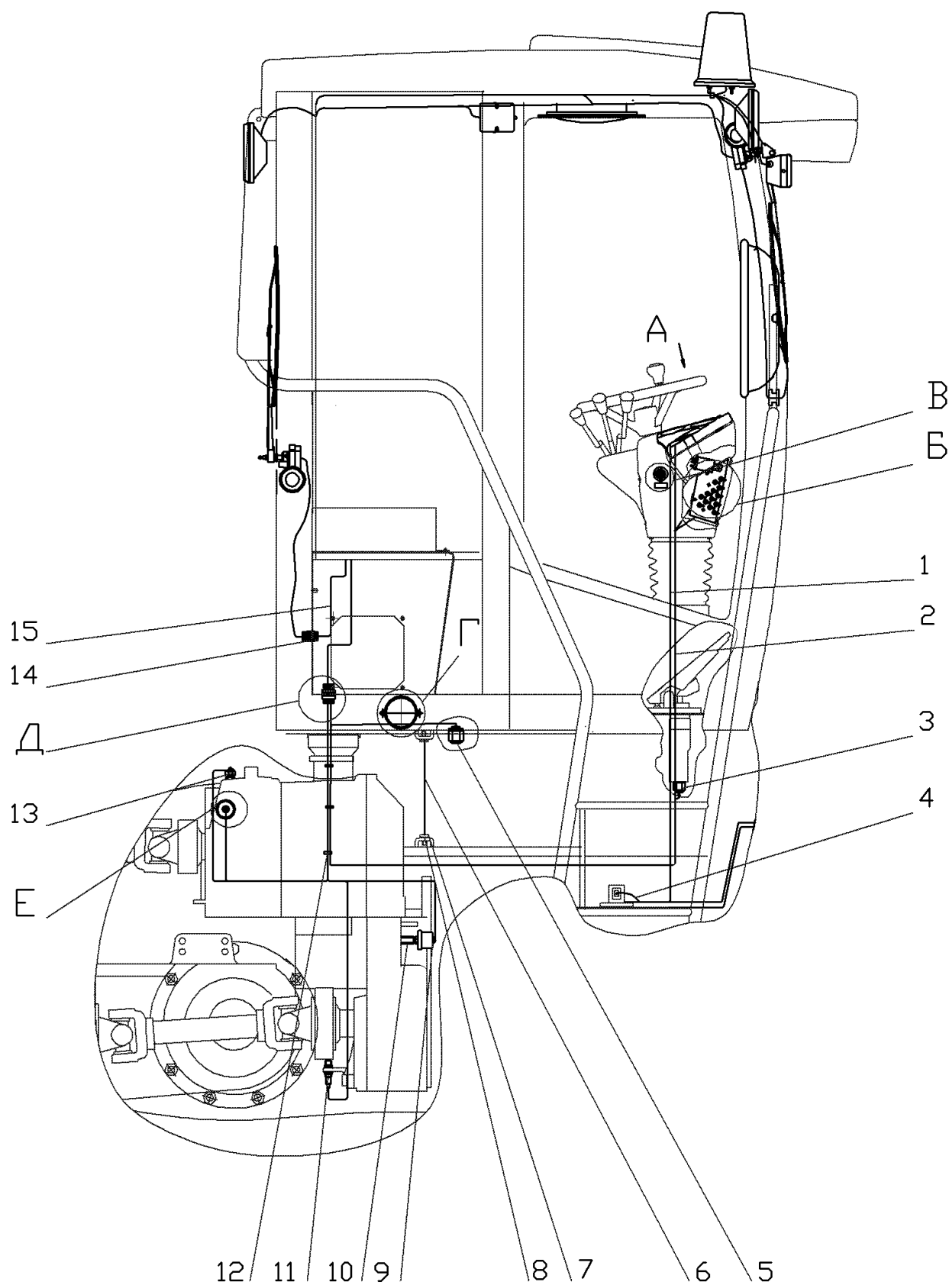
Рис. 40.6 Электрооборудование кабины
