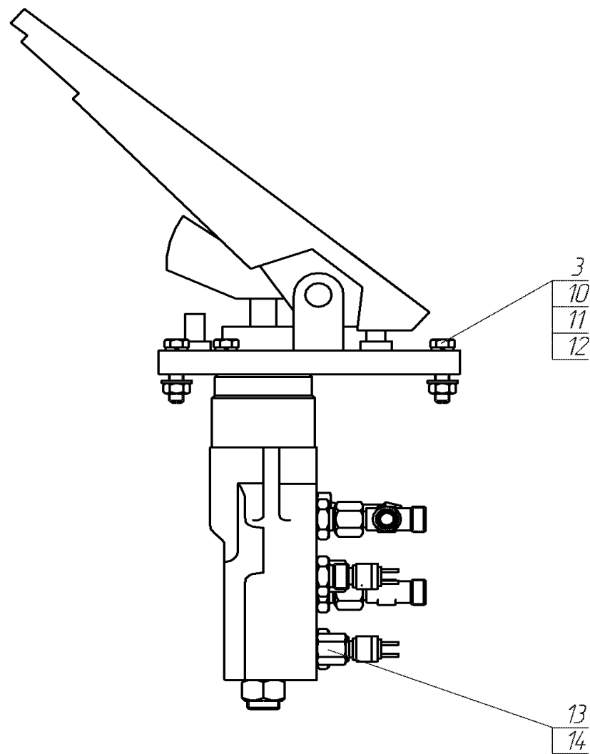
Рис. 36 Установка педали тормоза 257.11.01.00.000
