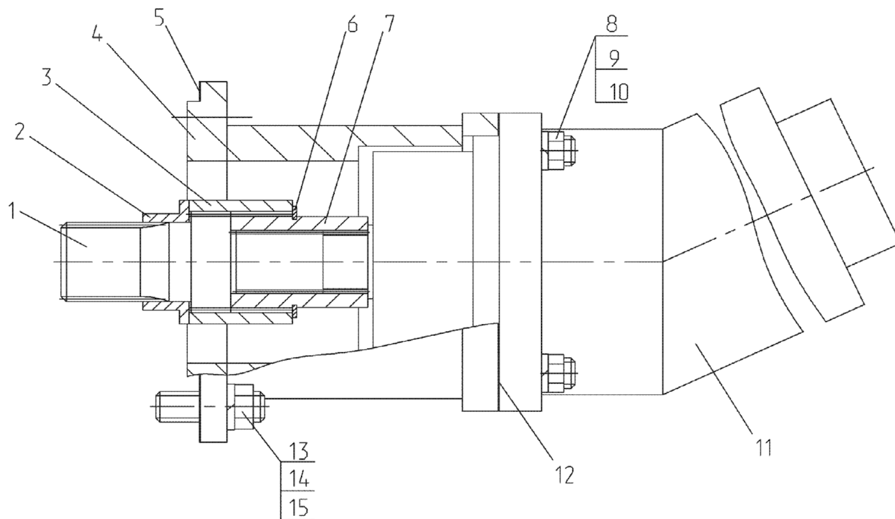
Рис. 53 Установка насоса 723.03.02.04.000
