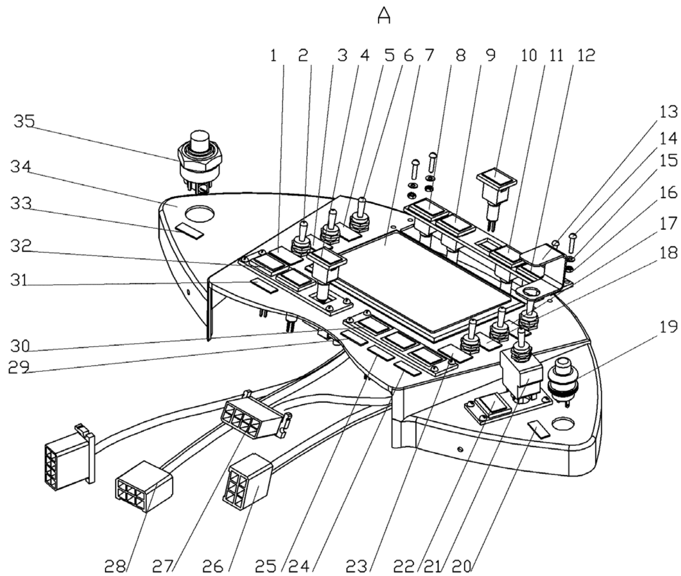
Рис. 40.7 Панель 724.09.08.00.000
