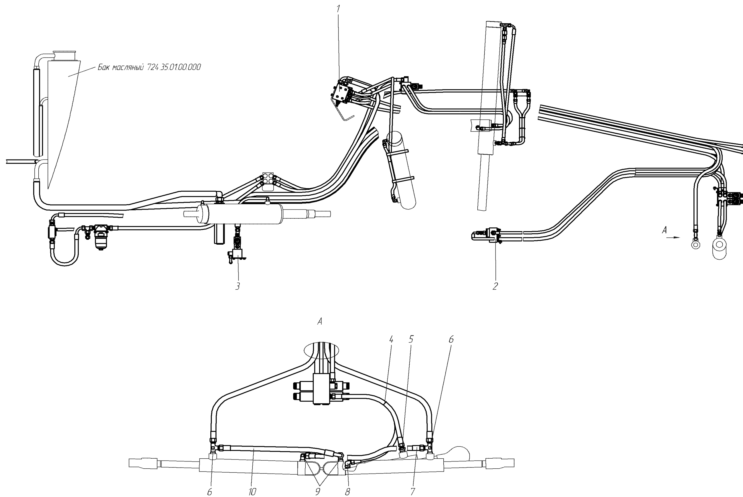
Рис. 30 Гидросистема 724.05.00.00.000
