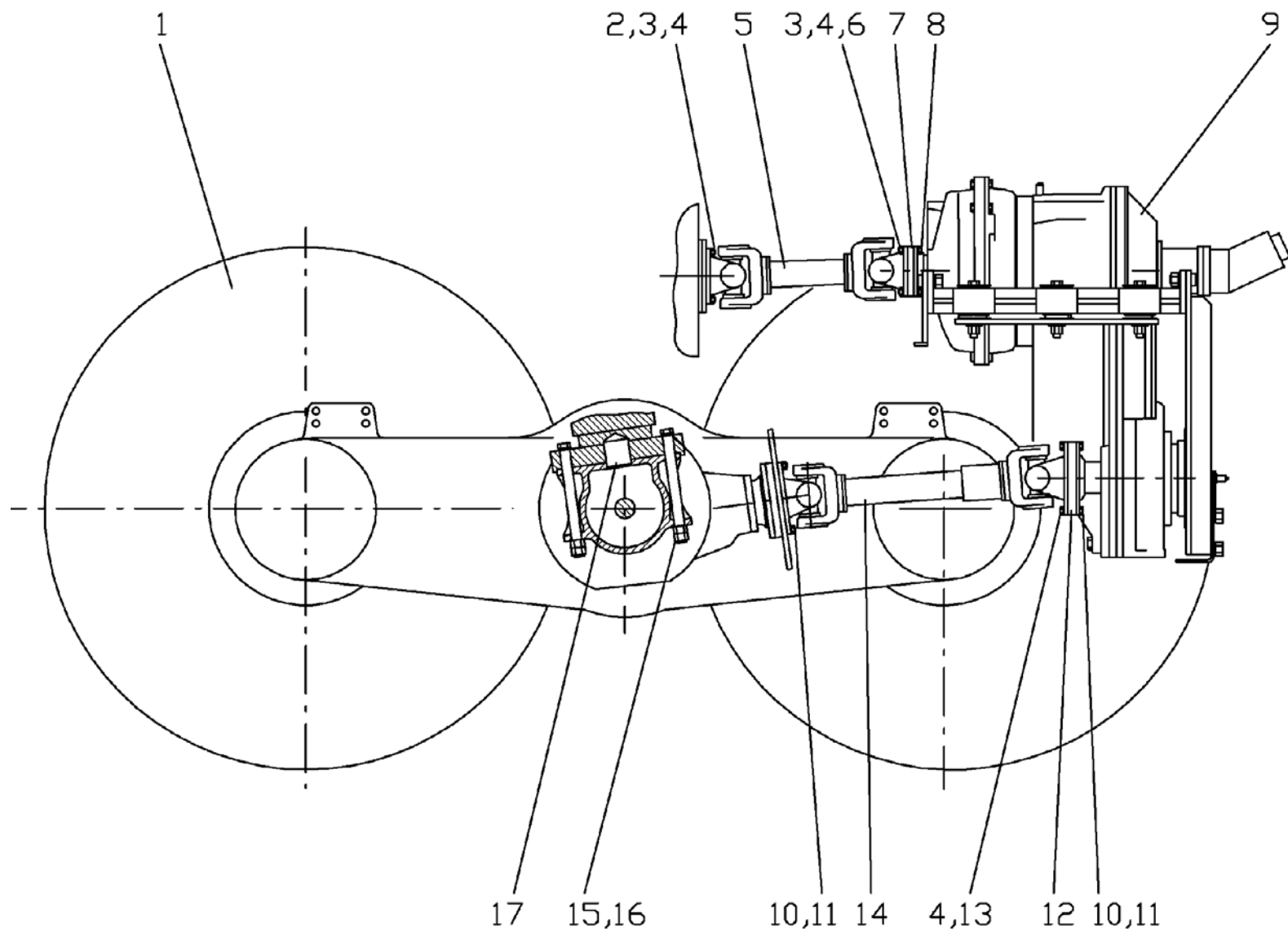
Рис. 50 Трансмиссия 724.03.00.00.000
