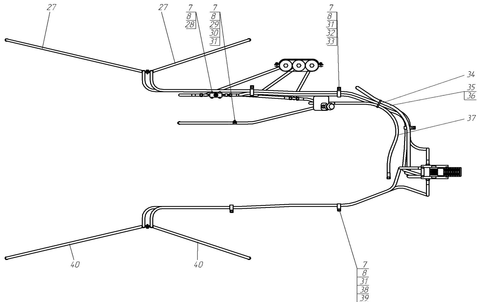
Рис. 35.2 Гидросистема тормозов 257.11.00.00.000
