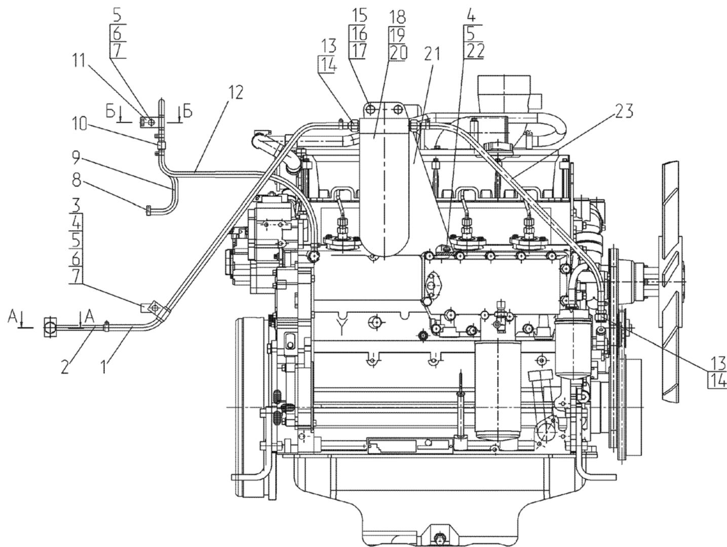
Рис. 48.1 Система питания 724.02.05.00.000
