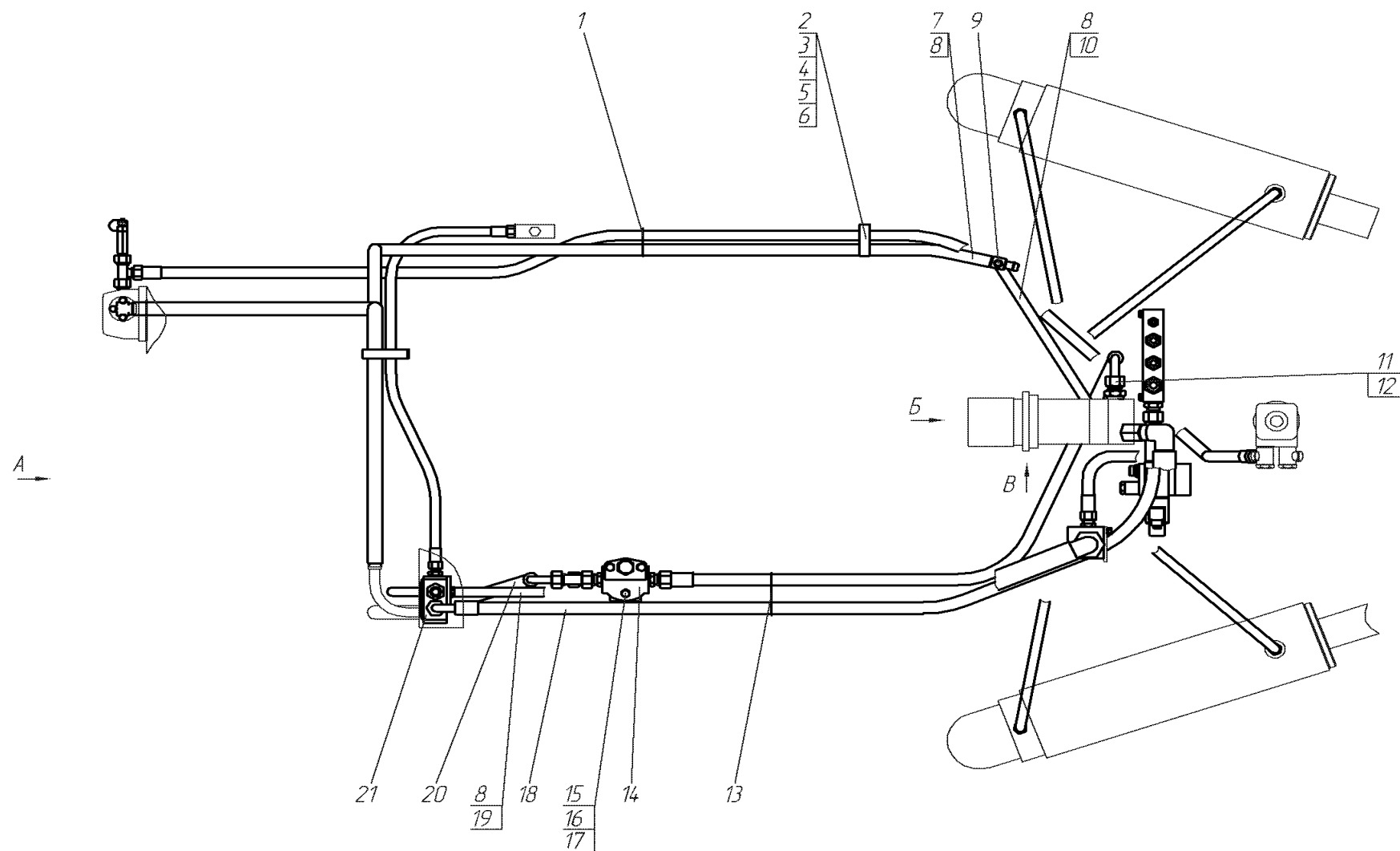
Рис. 31.1 Гидросистема рама подмоторной 724.05.01.00.000
