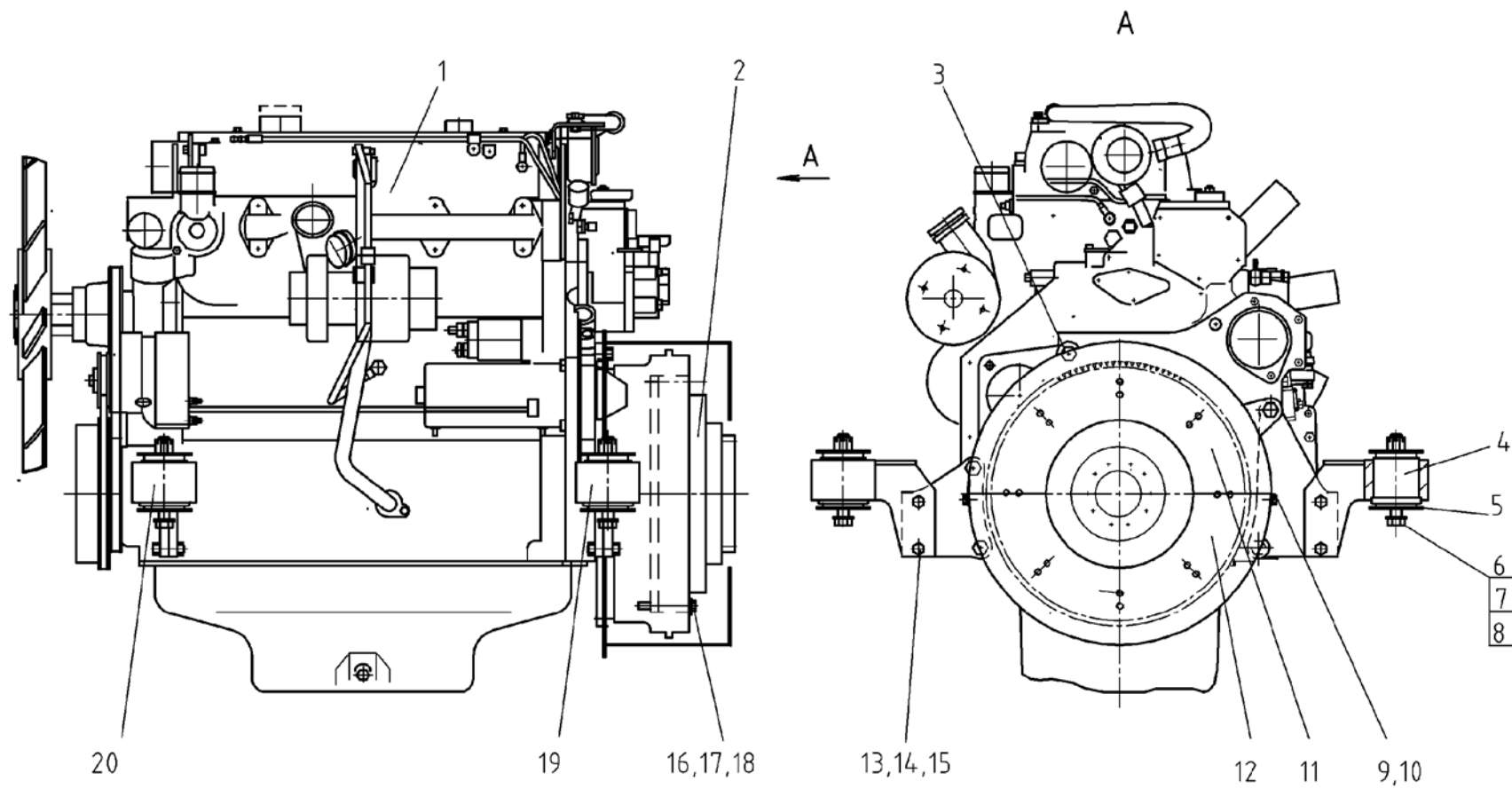
Рис. 42 Установка двигателя 724.02.01.00.000
