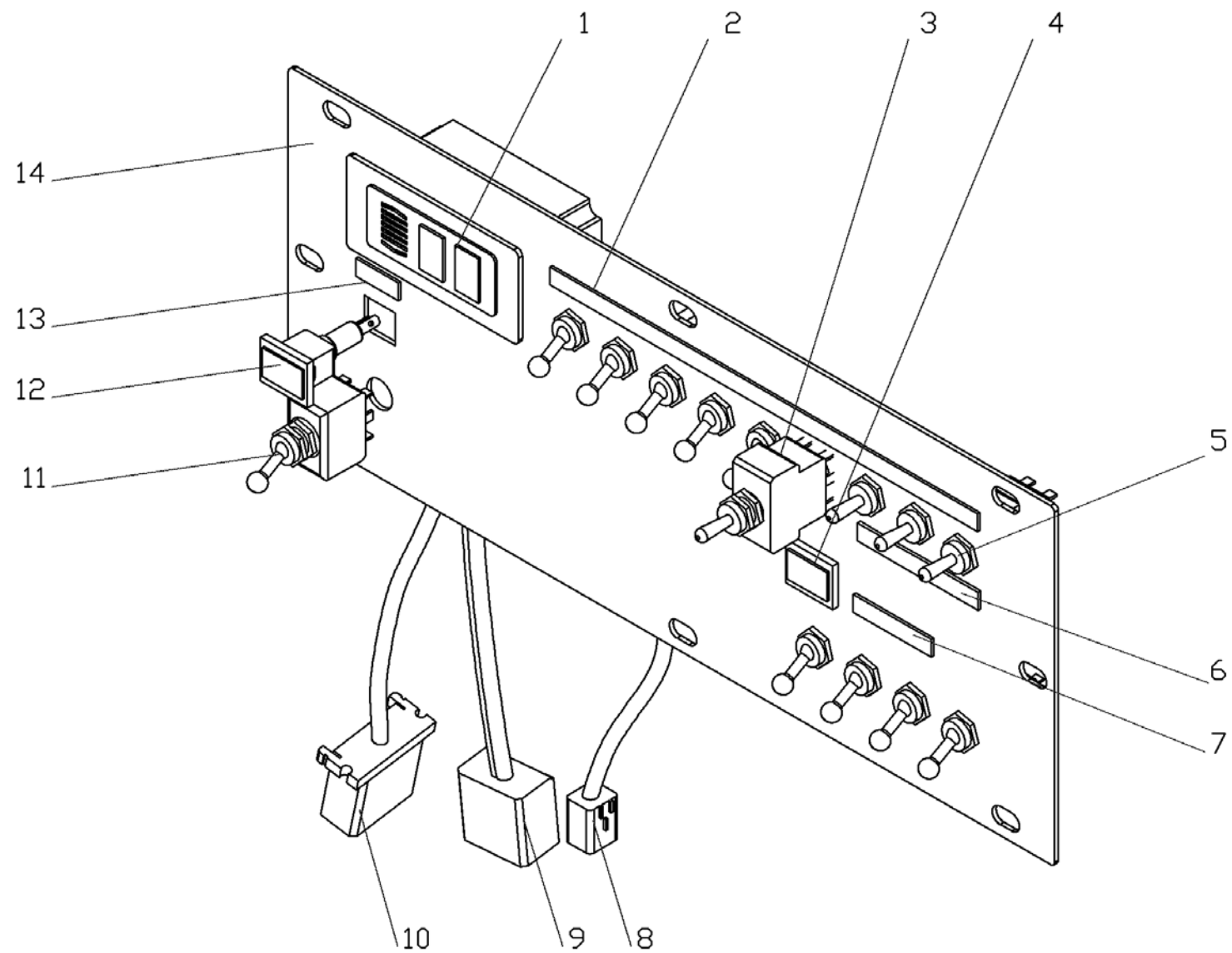
Рис. 40.11 Панель 751.09.02.00.000 - 116 -
